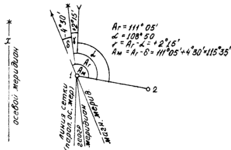
Рис.6 Схема углов точки 1
